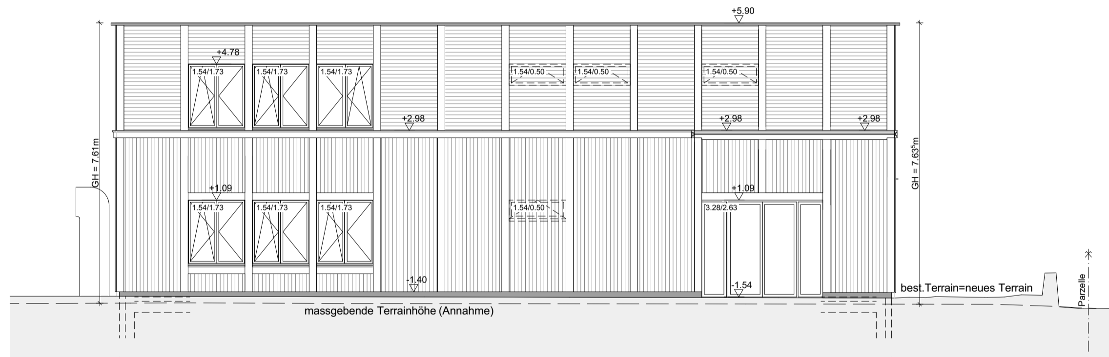
Nordfassade Neubau
