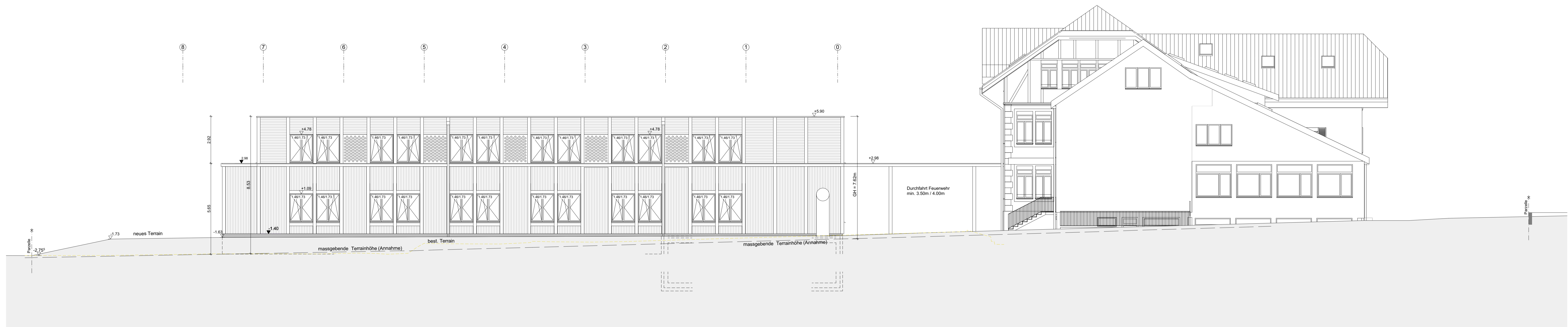
Ostfassade Neubau / Altbau
